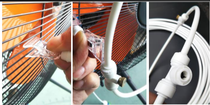
自在クリップで扇風機とホースを挟むだけ ホースを差し込む
